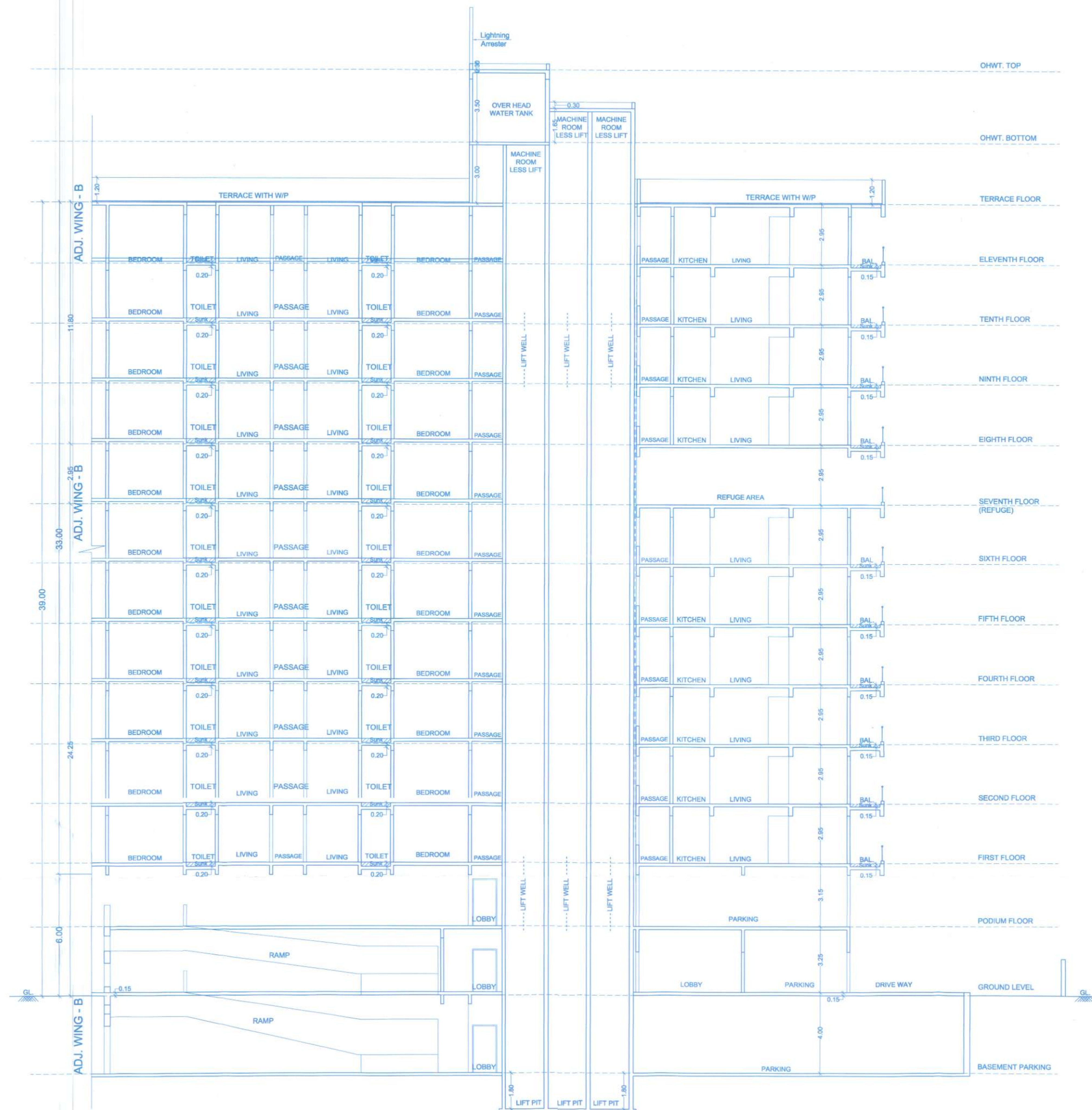
SECTION A-A SCALE 1:100
