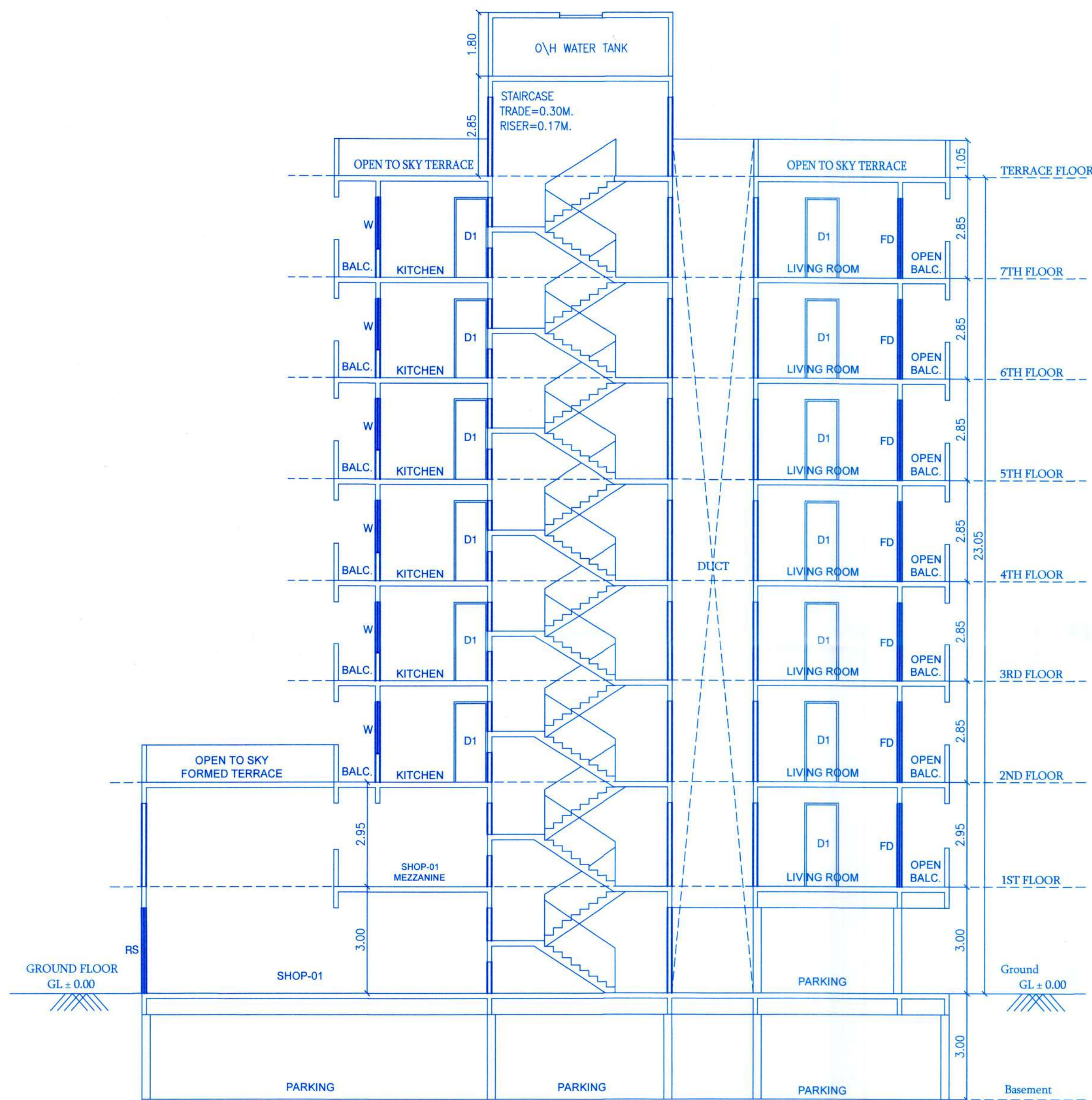
SECTION A-A
