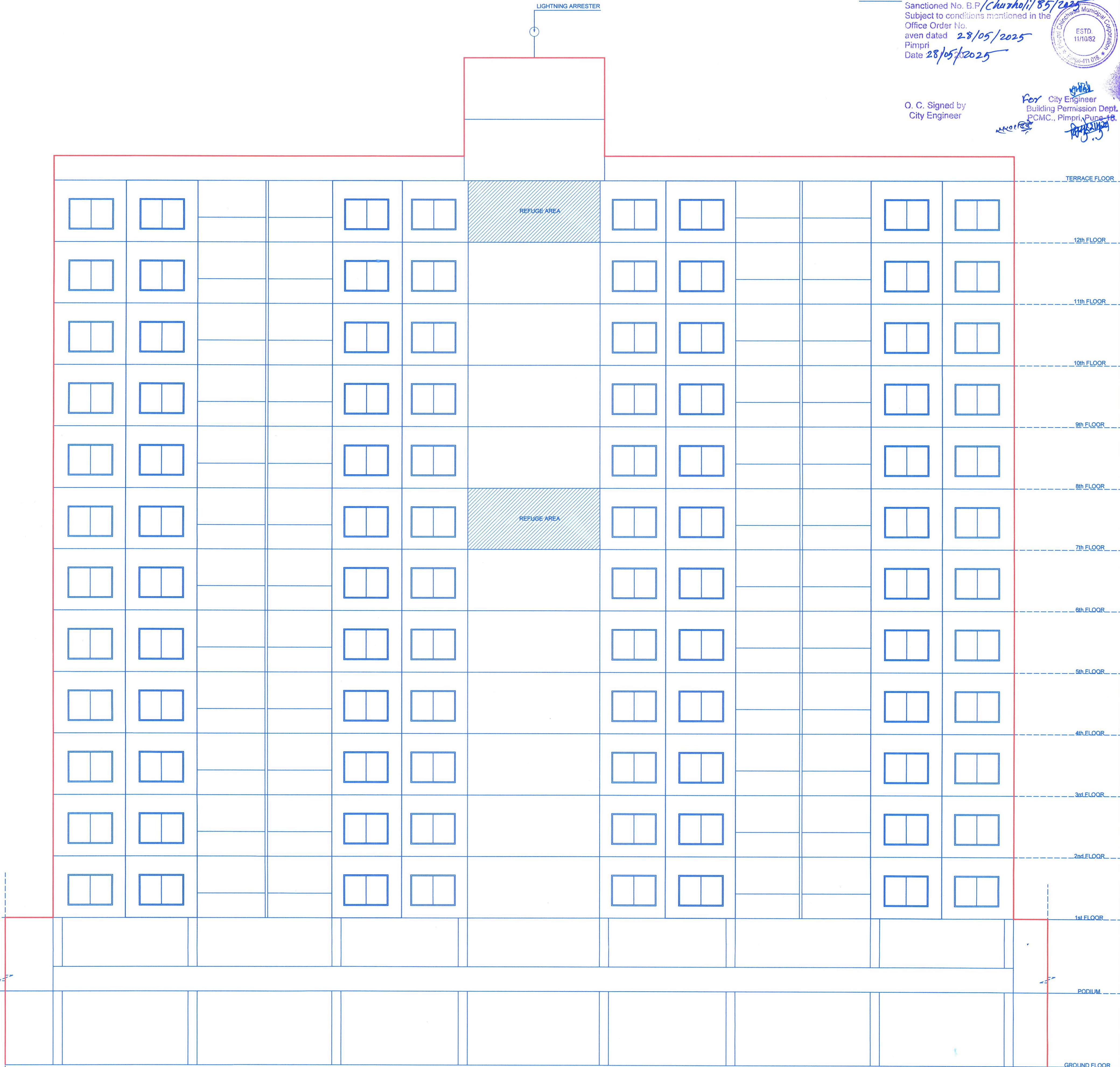
ELEVATION
